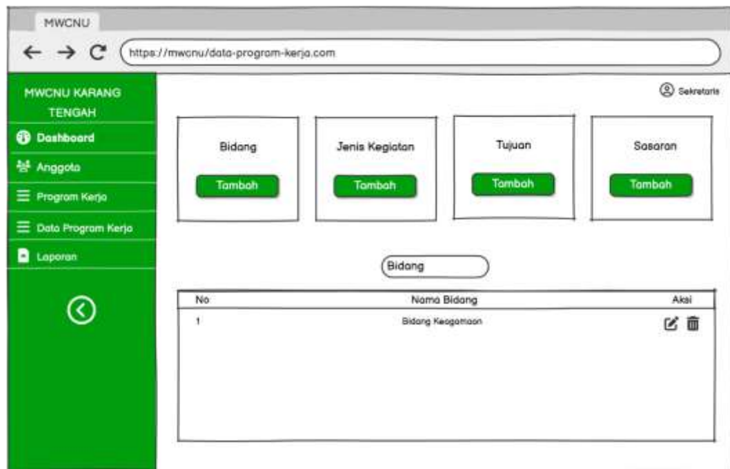
Gambar 4.79 Mockup Sekretaris Kelola Master Data Program Kerja
