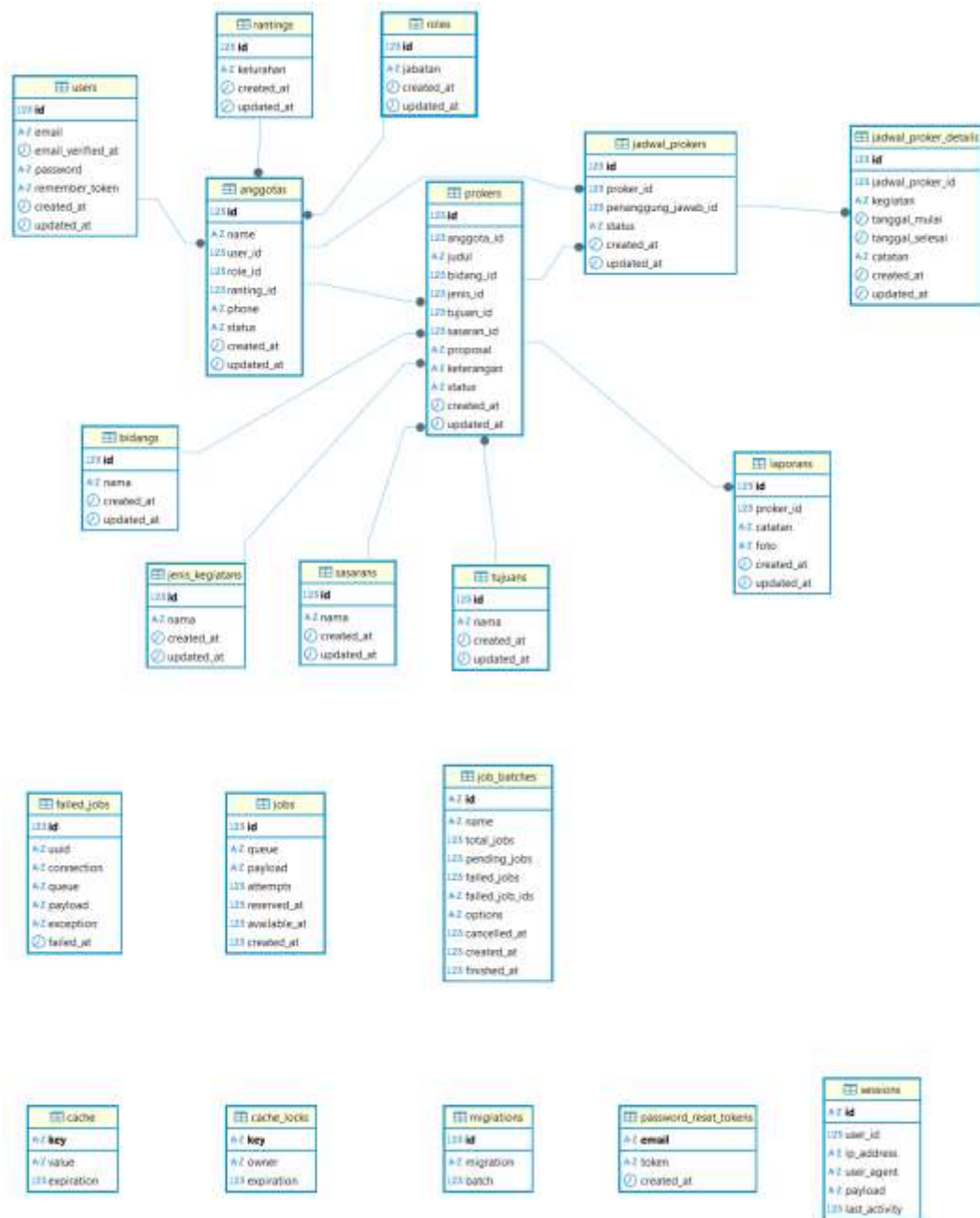
Gambar 4.53 Struktur Database
